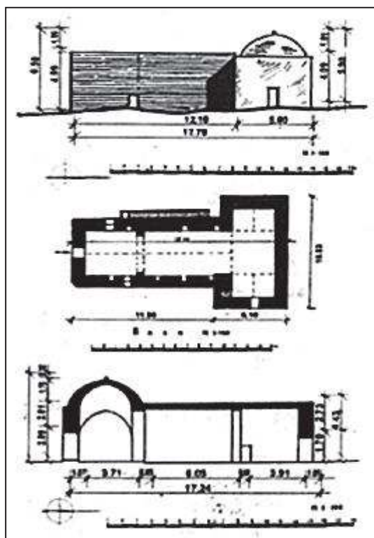
Tərəkmə məscidi. Ölçü və çertyoj Ş. Fətullayevindir.
